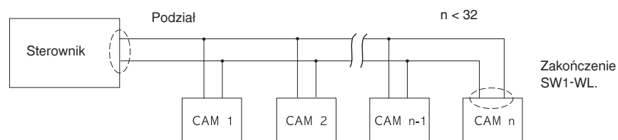
âOrganizacja półdupleksowa RS-485â
