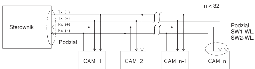
âOrganizacja pełnodupleksowa RS-422A/RS-485â
