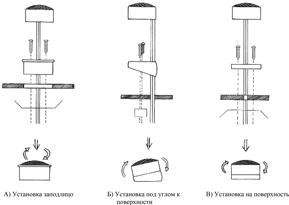
Рис. 1. Схема установки ВЧ-динамика.
