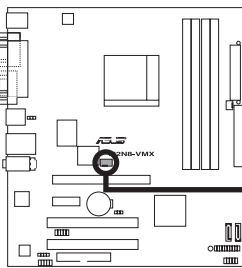
M2N8-VMX CPU Fan Connector
