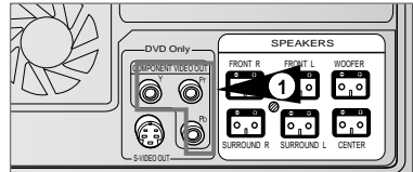
A TV Component Input bemenetéhez
