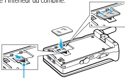
Dispositif de fixation de la carte SIM
